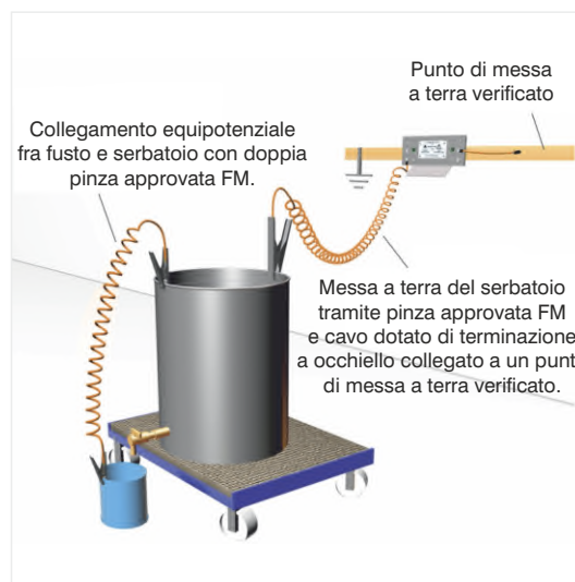
Cen-Stat™ cable
