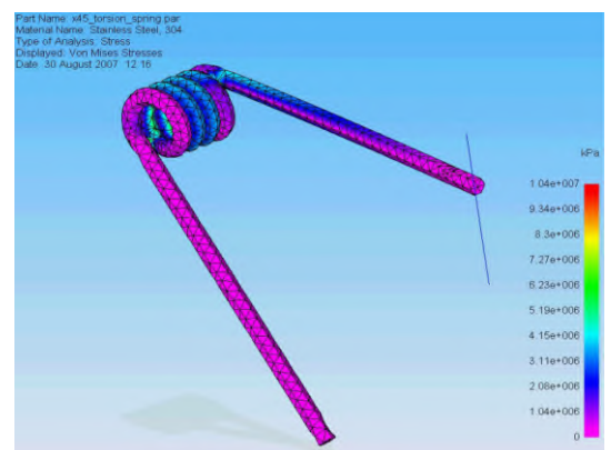
Le molle di Newson Gale sono progettate e analizzate con l'ausilio della tecnologia dell'analisi degli elementi finiti.
